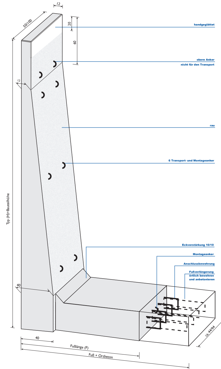
Typ 555 - 605 mit Anschlussbewehrung
