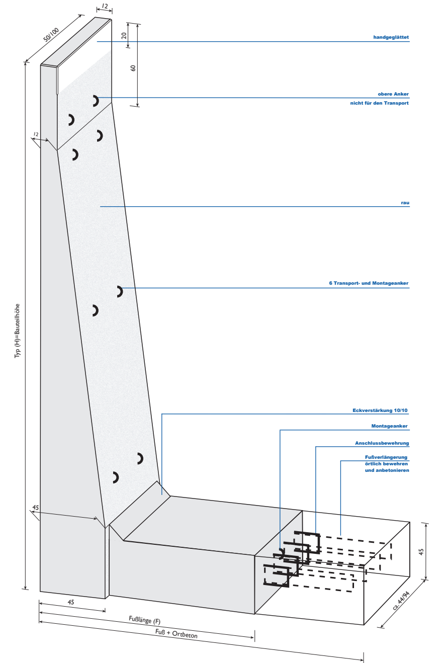
Typ 630 - 655 mit Anschlussbewehrung
