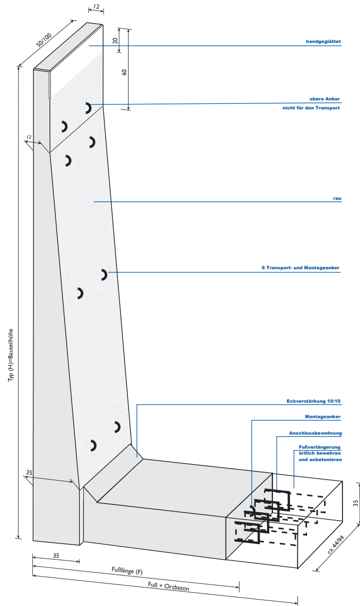
Typ 480 - 530 mit Anschlussbewehrung
